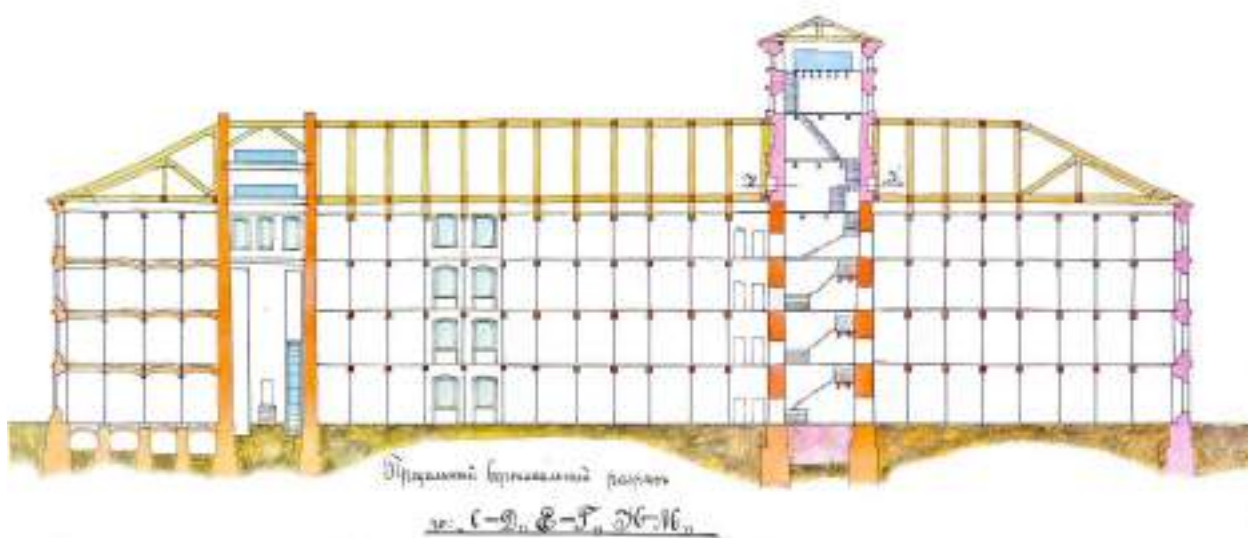
Рис. 5. Продольный разрез прядильного корпуса. Архивный чертеж 1895 г.
