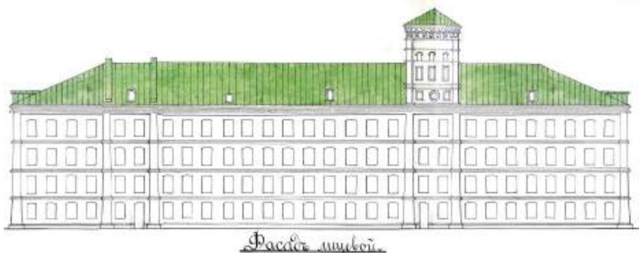
Рис. 8. Северный фасад прядильного корпуса. Архивный чертеж 1895 г
