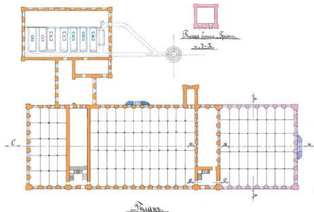
Рис. 6. План прядильного корпуса. Проект пристройки справа (выделена розовым цветом стен) и надстройки гринельной башни. Архивный чертеж 1895 г.
