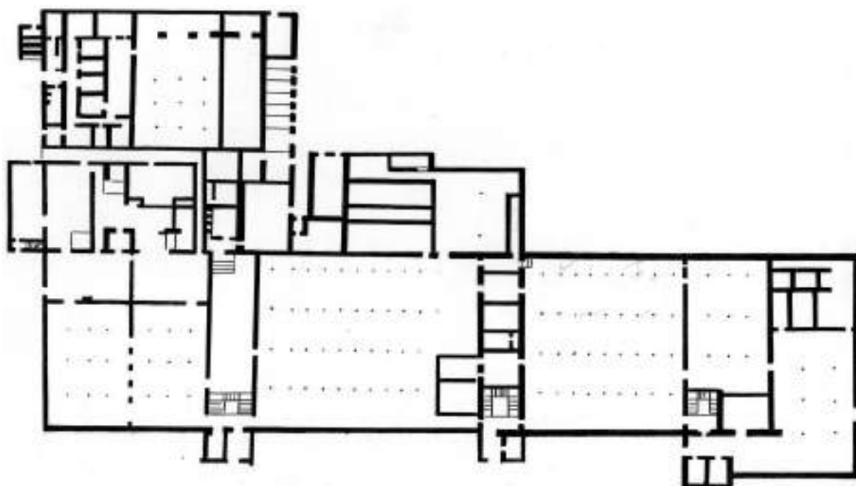
Рис. 7. Схема прядильного корпуса. Современное состояние
