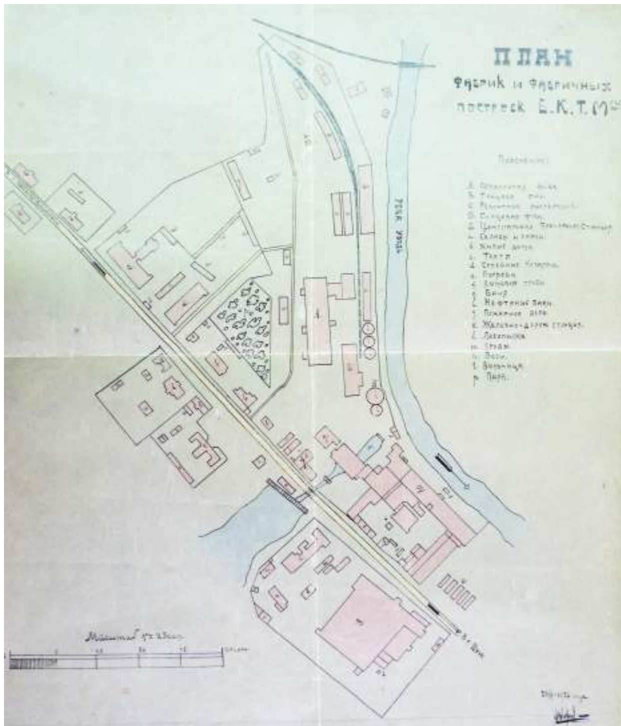
Рис. 4. Генеральный план Большого Кохомского товарищества мануфактур. Архивный чертеж 1926 г.
