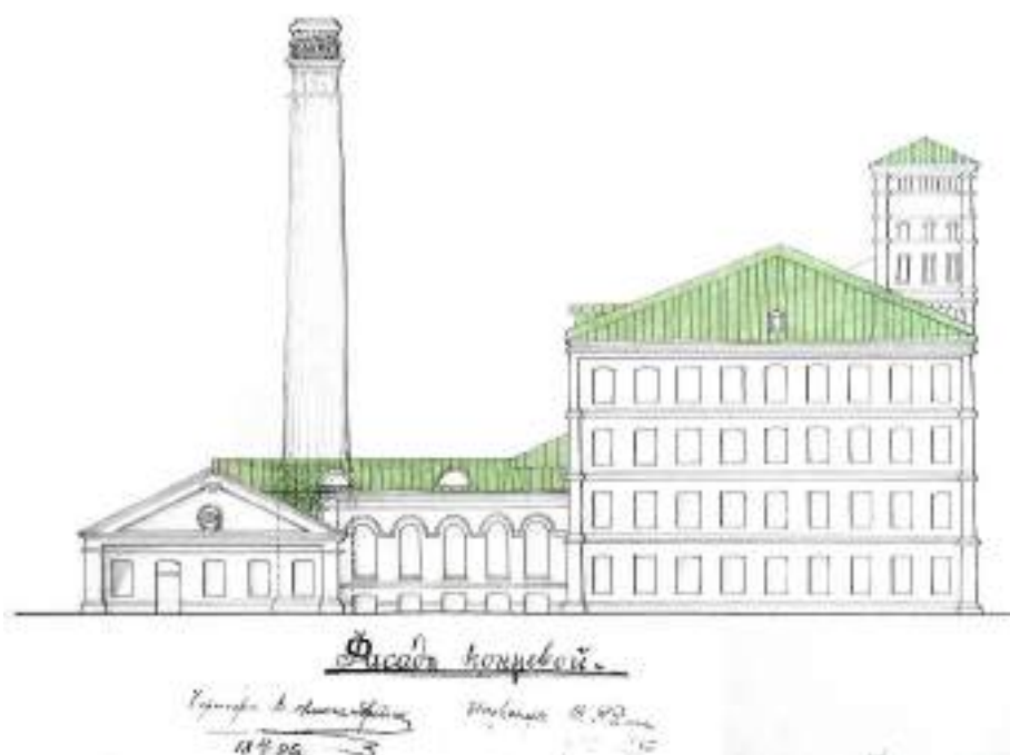
Рис. 8. Северный фасад прядильного корпуса. Архивный чертеж 1895 г
