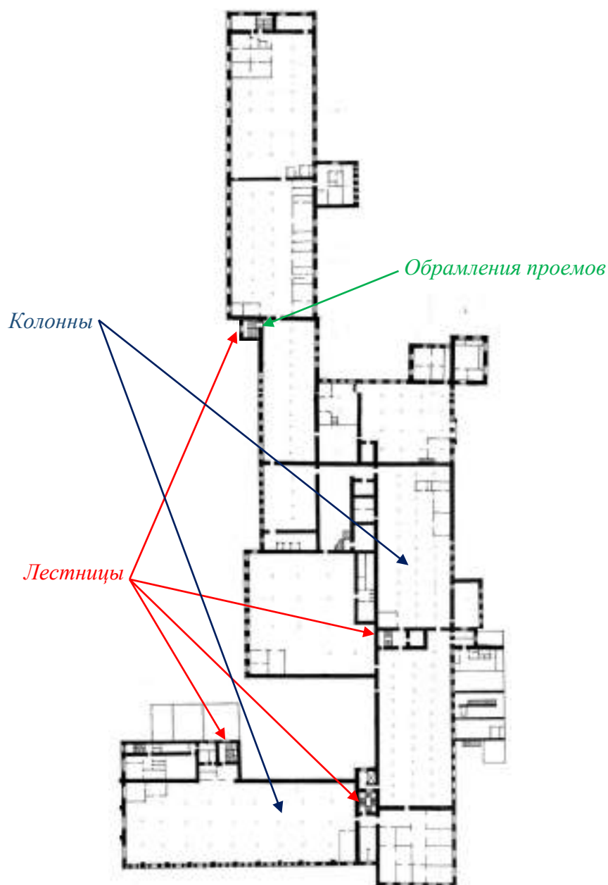
Рис.90. Схема расположения ценных элементов интерьеров отделочного корпуса
