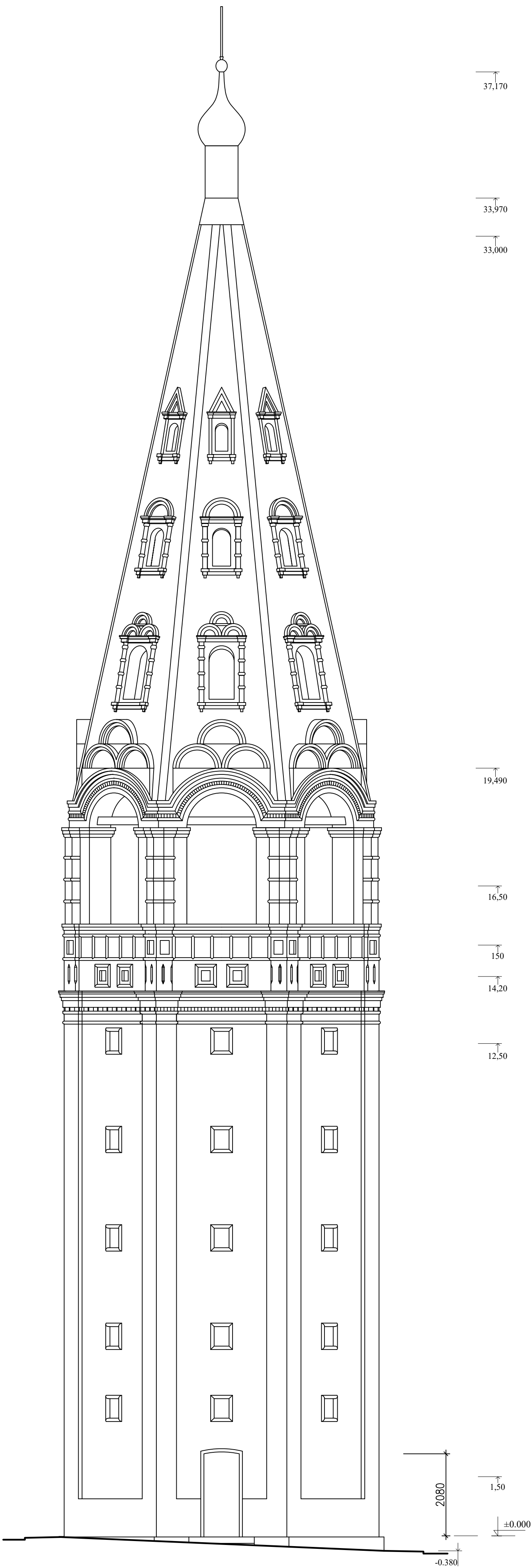
Северный фасад
