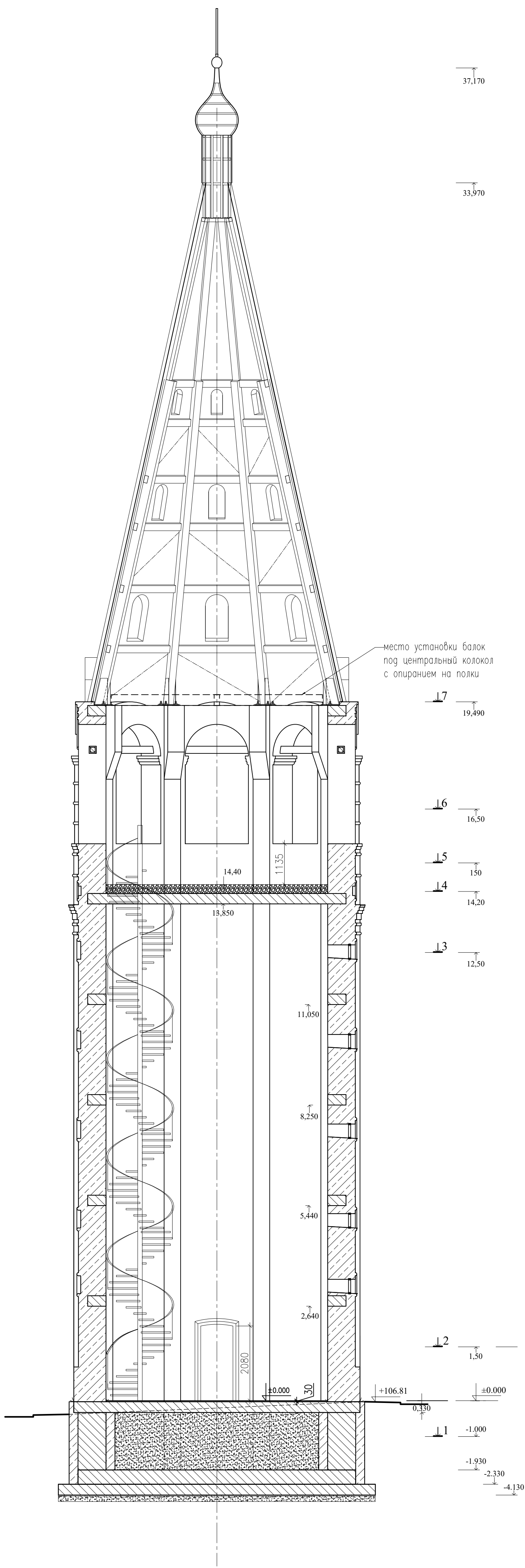
Разрез 1 - 1
