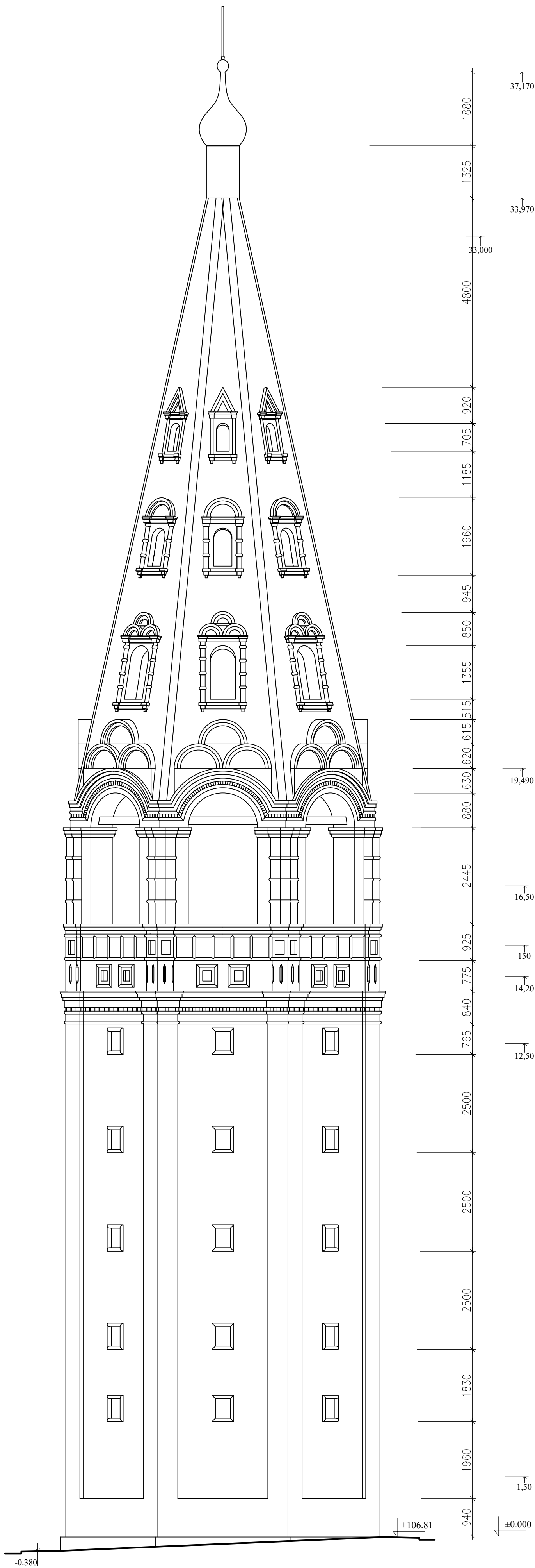
Южный фасад.
