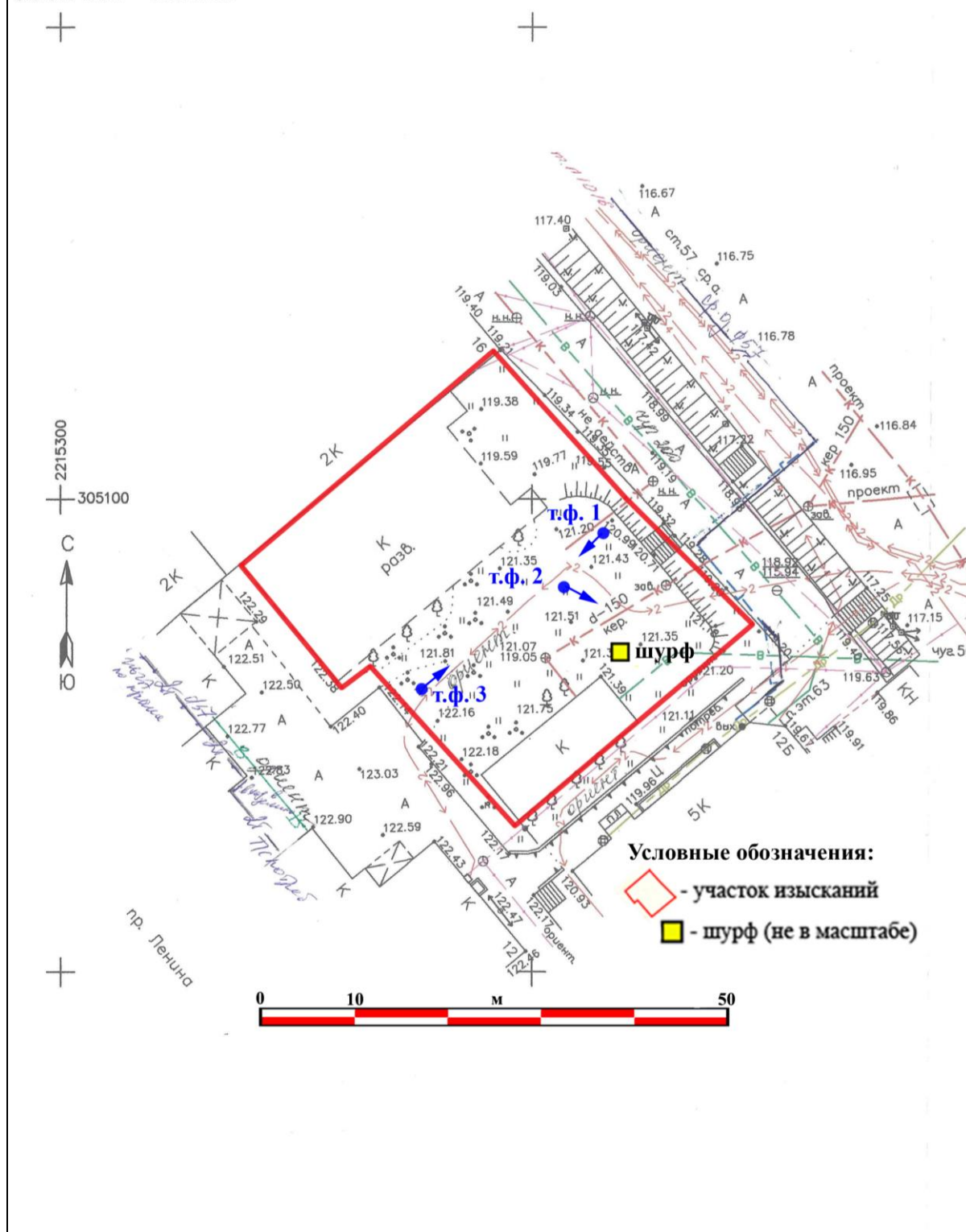
Рис. 11. г. Иваново, пр. Ленина, 12А, участок к/н 37:24:010109:183. Участок проведения работ, топографический план (документация заказчика).
