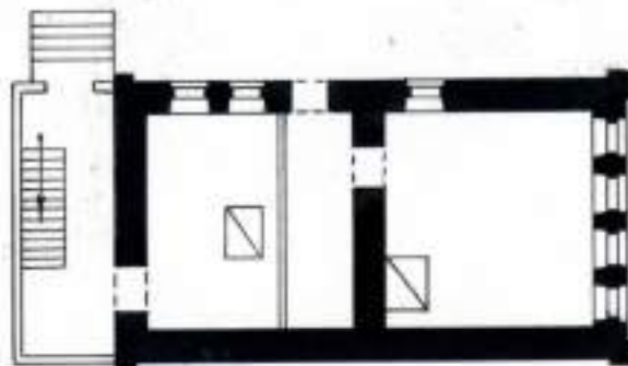
План I этажа
