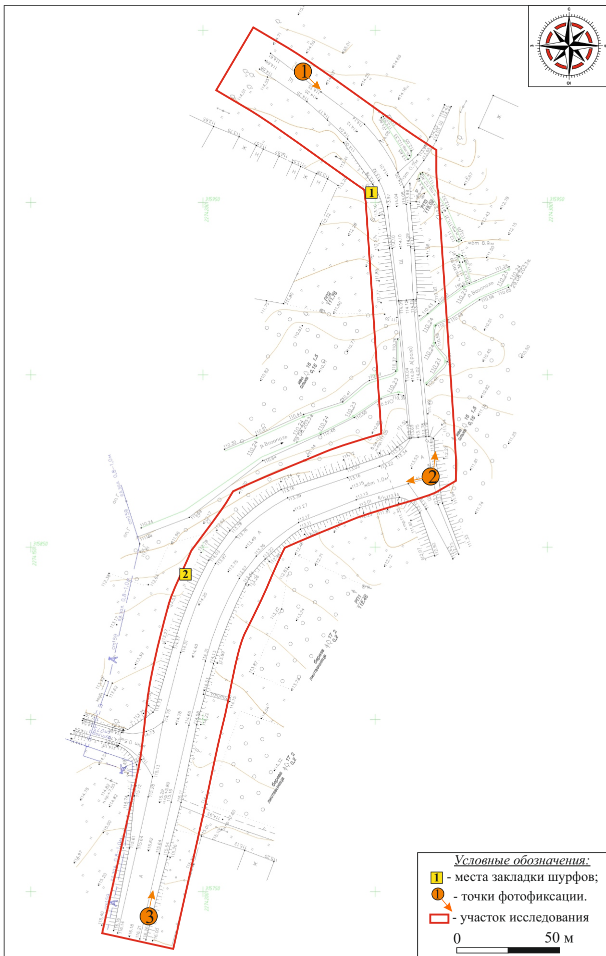
Илл. 7. Ивановская область, Родниковский район, с. Филисово, реконструкция моста через реку Возополь - 2023 г. Топоплан участка исследования с расположением шурфов и точек фиксации (топооснова предоставлена Заказчиком).
